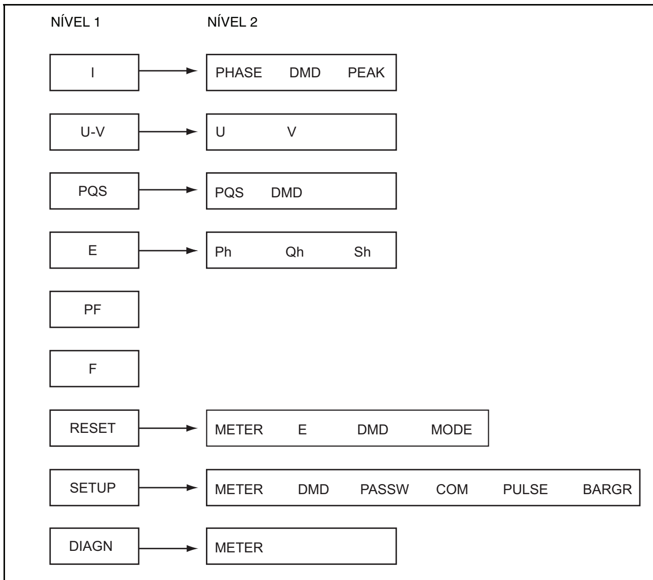
Figura 6–2: Lista abreviada de itens de menu do medidor de energia elétrica IEC
